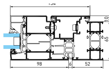
Ouvrant Apparent châssis basculant-pivotant
